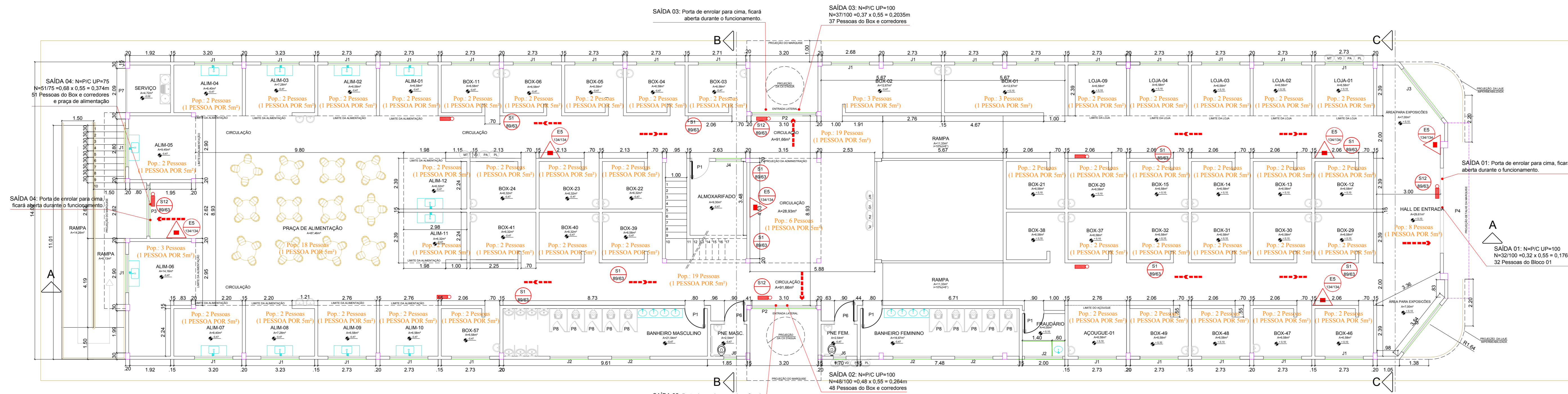
PLANTA BAIXA PAVIMENTO TÉRREO ESCALA 1/100
