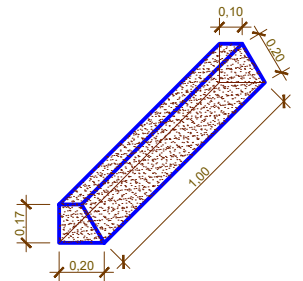
PROJETO MEIO FIO SEM SARJETAS( Com Máquinas) ( 0,024 M 2 / ML)
